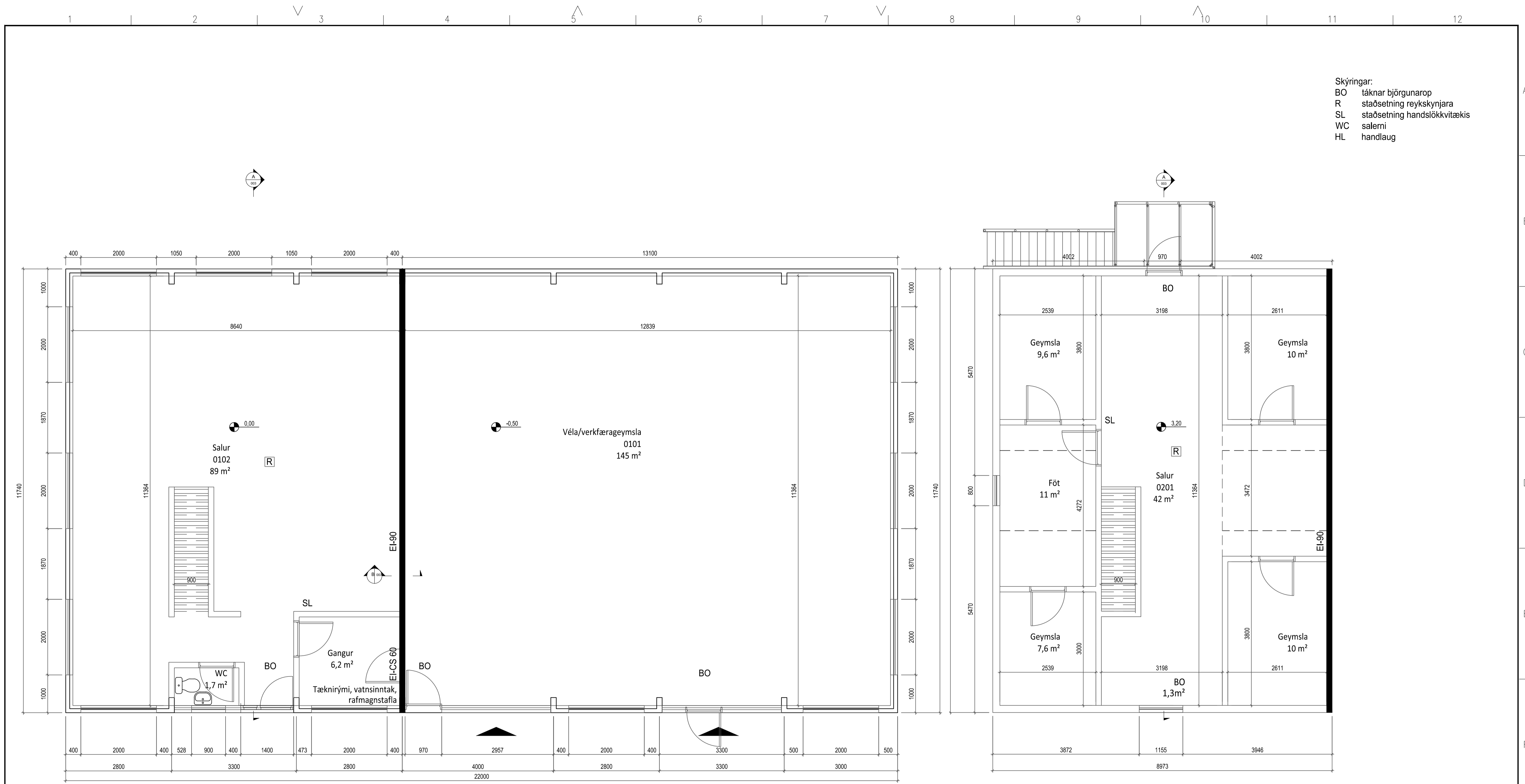
GRUNNMÝND 1. HÆÐ 1:50
